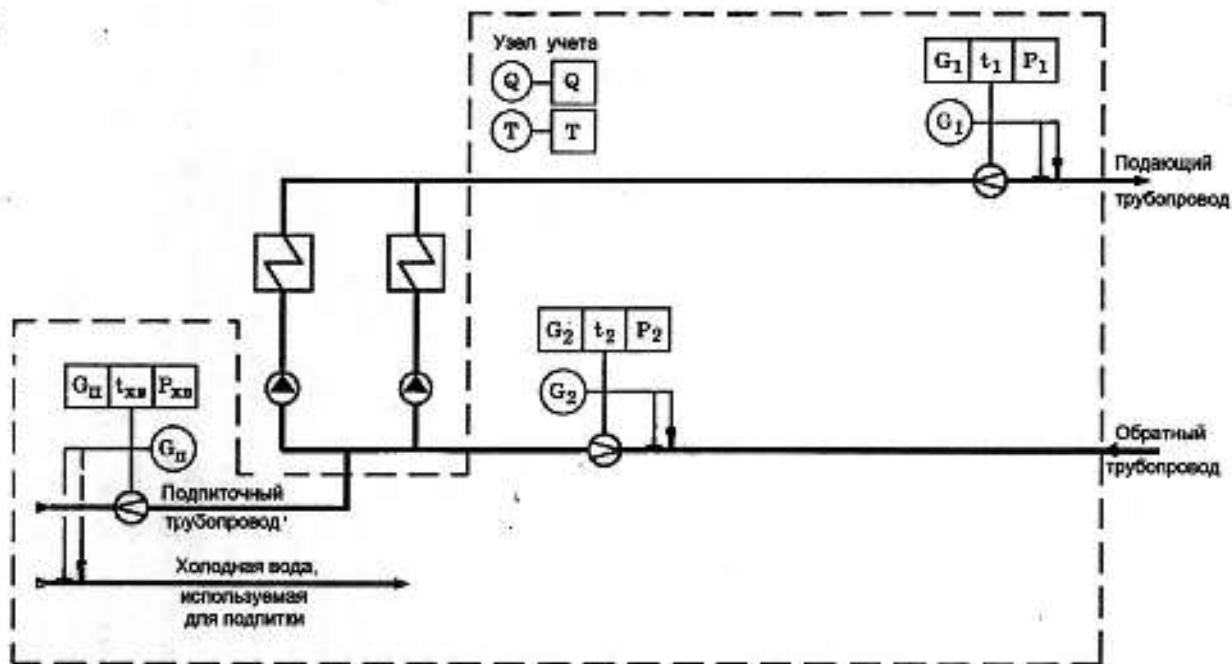
Рис. 1. Принципиальная схема размещения точек измерения массы (объема) теплоносителя и его регистрируемых параметров на источнике теплоты для водных систем теплоснабжения
