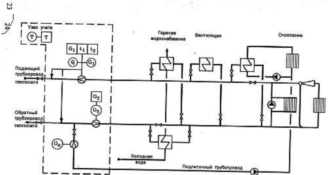
Рис. 4. Принципиальная схема размещения точек измерения количества тепловой энергии и массы (объема) теплоносителя, а также его регистрируемых параметров в закрытых системах теплоснабжения
